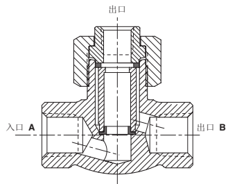
6330 系列: 旁通式过滤器
