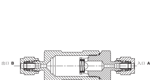
6310 系列: 管道在线式过滤器
