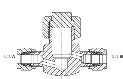
6320 系列: 可拆卸式过滤器
