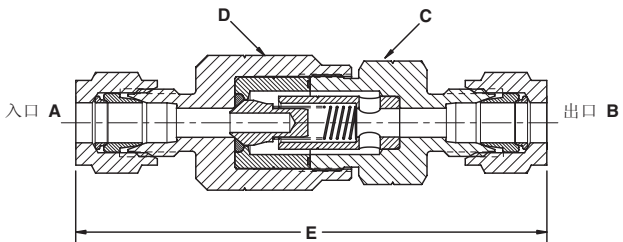
6200 系列提升式止回阀
