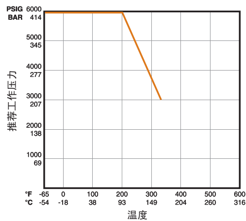
压力与温度
