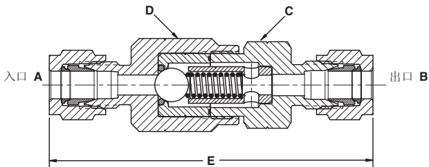
6100 系列球型止回阀
