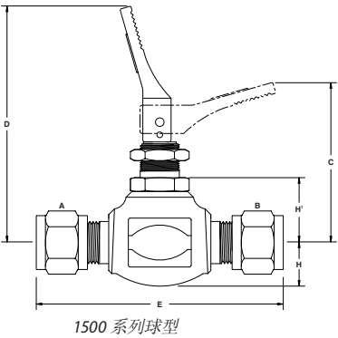
1500 系列球型
