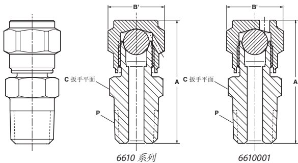
6610 系列: 直型阀
