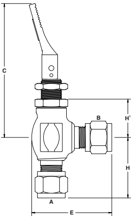
1500 系列角型
